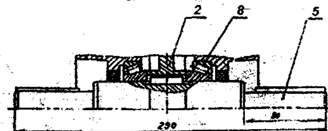
Рис. 8. Вариант сборки 56. Остальное - см. рис. 1
