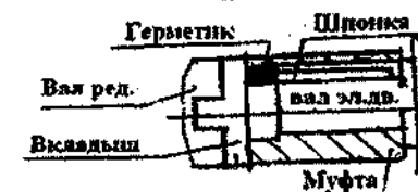
Рис. 9а Герметизация шпоночного паза.
