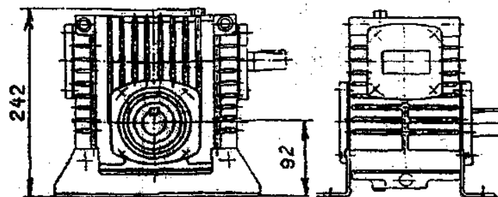
Рис. 3. Конструктивное исполнение по способу монтажа 1211. Остальное - см. рис. 1
